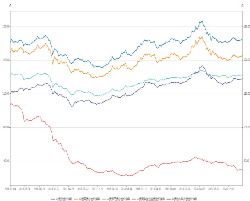
图 3: 国内债市
