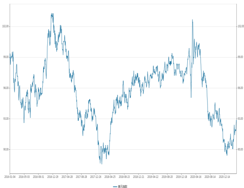
图 5: 美元指数
